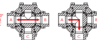
VÁLVULA DE ESFERA TRIPARTIDA PASSAGEM REDUZIDA (PR)
