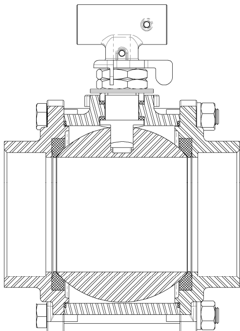
Figura 1 – Corte transversal da VET 4"PP S1000 Cl. 300 Montada.
