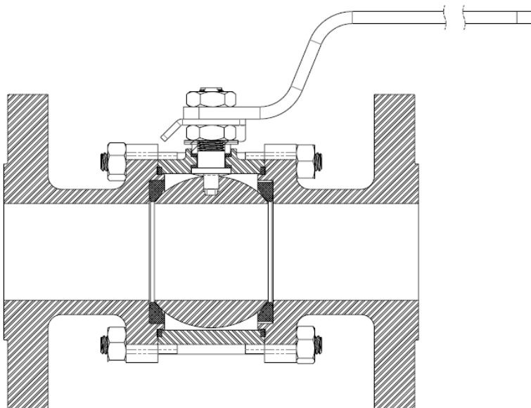
Figura1 – VET Flange S1000 Classe 300.
