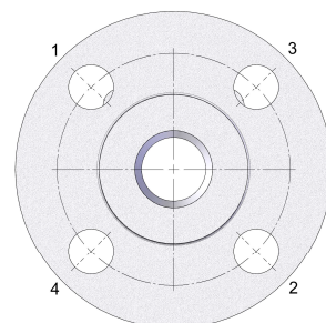
Figura2 – Seqüência de aperto dos parafusos Flange
